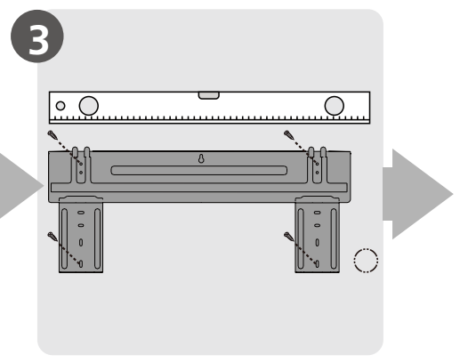
3 Befestigen der Montageplatte
