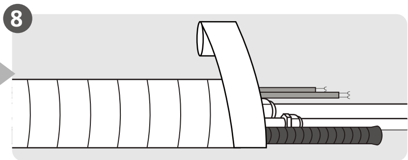
8 Ummantelung von Leitungen und Kabeln (gilt nicht für einige Standorte in den USA)
