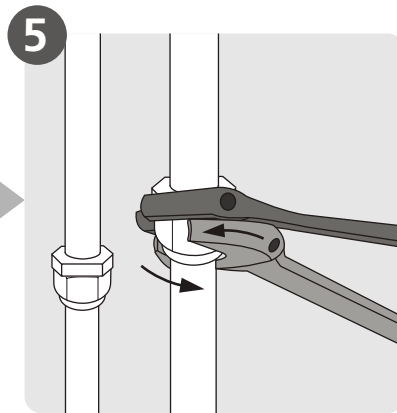
5 Die Rohre anschließen
