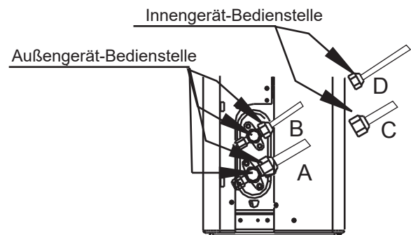
An: Niederdruck-Absperrventil B: Hochdruck-Absperrventil C&D: Bördelmuttern für Innengerät
