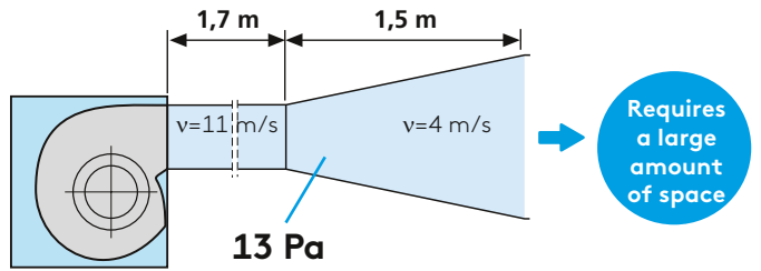
Airflow 4 m³/s
