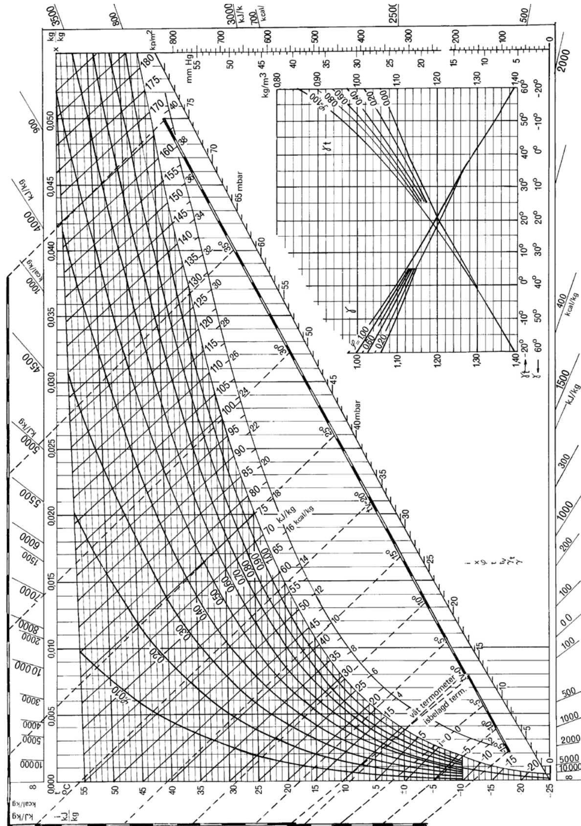
Mollier diagram for humid air -25 till +55 °C
