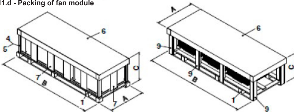
Fig.11.d - Packing of fan module
