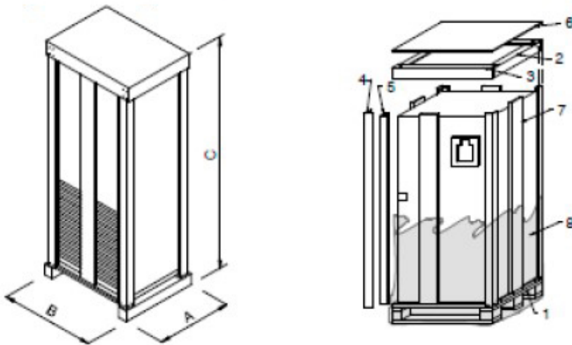
Fig.11.d - Packing of fan module
